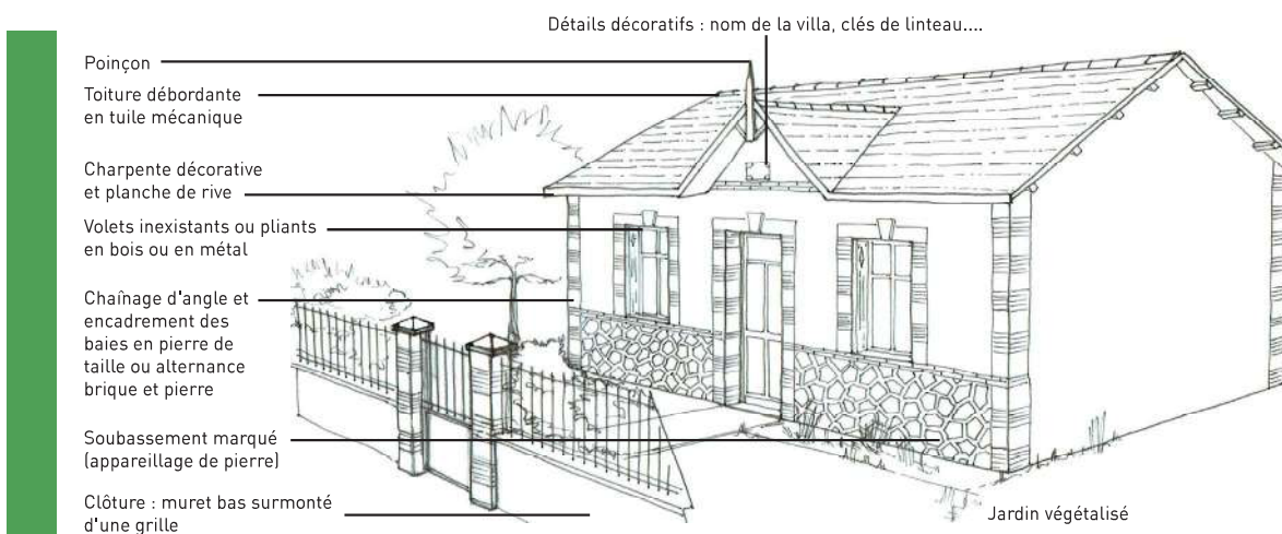
Une maison basse à fronton et ses caractéristiques
