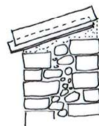
Couronnement d'un mur en tuile
