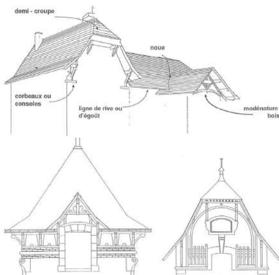
Divers débords de toiture et charpentes ornementées
