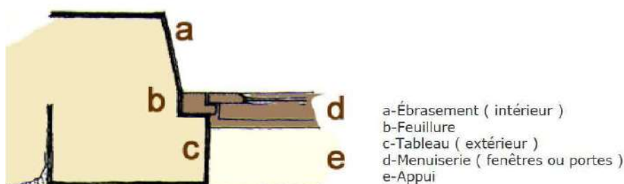
Schéma d'une baie - pose en feuillure Source : UDAP 17
